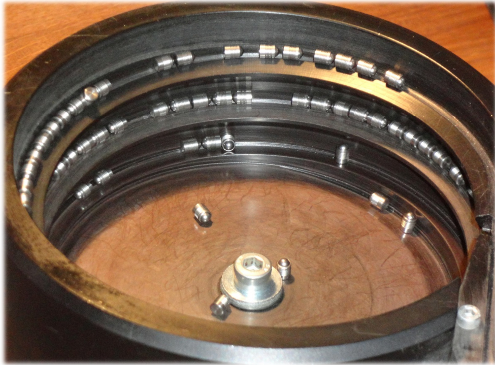
Zuführung Kugeldichtstopfen \varnothing 5 mm
