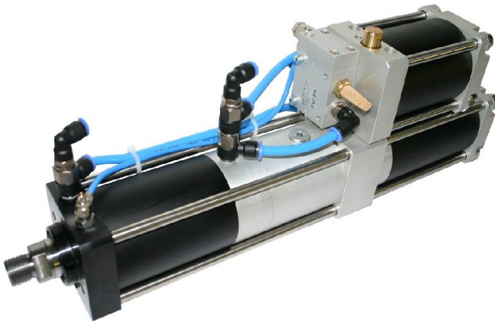
Powerzylinder, 100 mm Gesamthub, 6 mm Krafthub, 13 kN bei 6 bar
